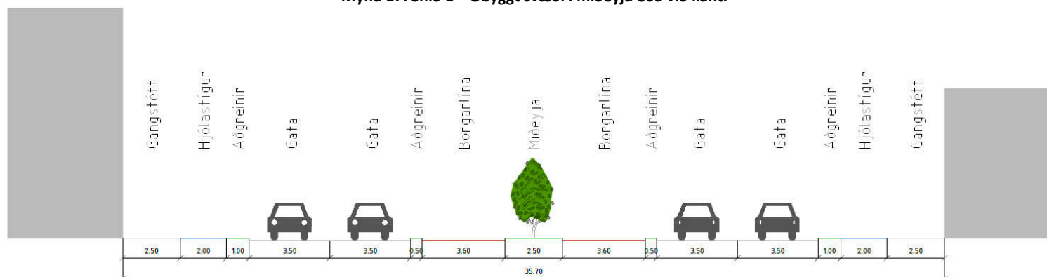
Mynd 18: Dæmi um snið fyrir 2 akreinar Borgarlínu og 4 almennar akreinar í götu í þéttbýli með 50 km/klst hámarkshraða.
