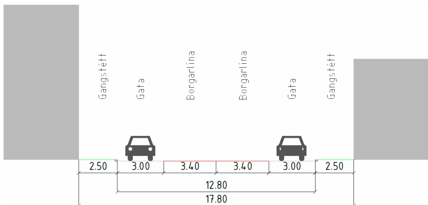
Mynd 8: Helstu stærðir í sniði fyrir 2 akreinar Borgarlínu og 2 almennar akreinar í götu á þéttbýli með 30-40 km/klst hámarkshraða.
