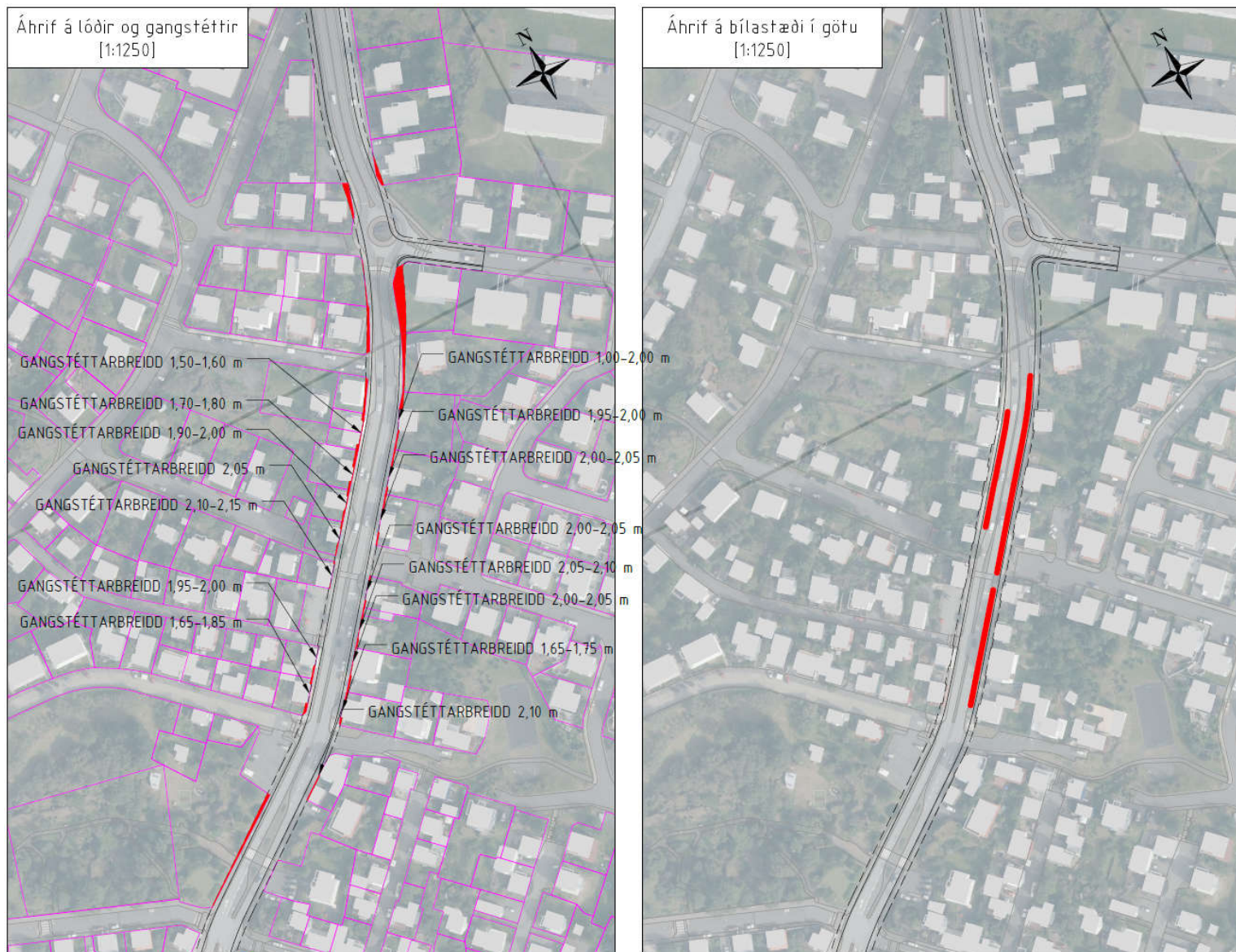
Mynd 14: Áhrif á lóðir og gangstéttbreiddir (vinstri) og bílastæði (hægri) (rauðar línur sýna bílastæði sem þyrftu að víkja) ef 4 akreina sniði er komið fyrir.
